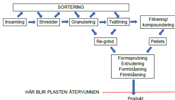
Figur 6: Processteg för mekanisk återvinning av plast. 45
