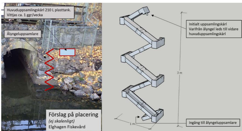
Figur 35. Förslag på placering och typ av ålyngeluppsamlare vid Uddby kraftverk. Elghagen fiskevård 2017.
