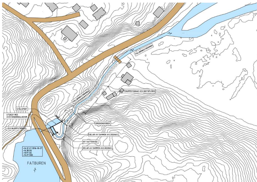
Figur 29. Översikt över föreslagna naturliknande fiskväg vid Fatbursdammen, PLAN. Norconsult 2017.
