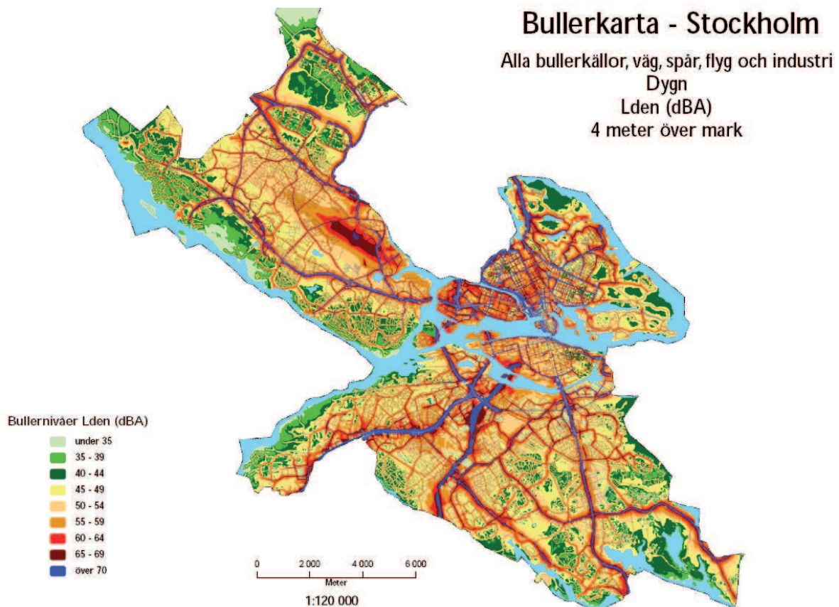
Figur 17 Bullerkarta - Stockholm
