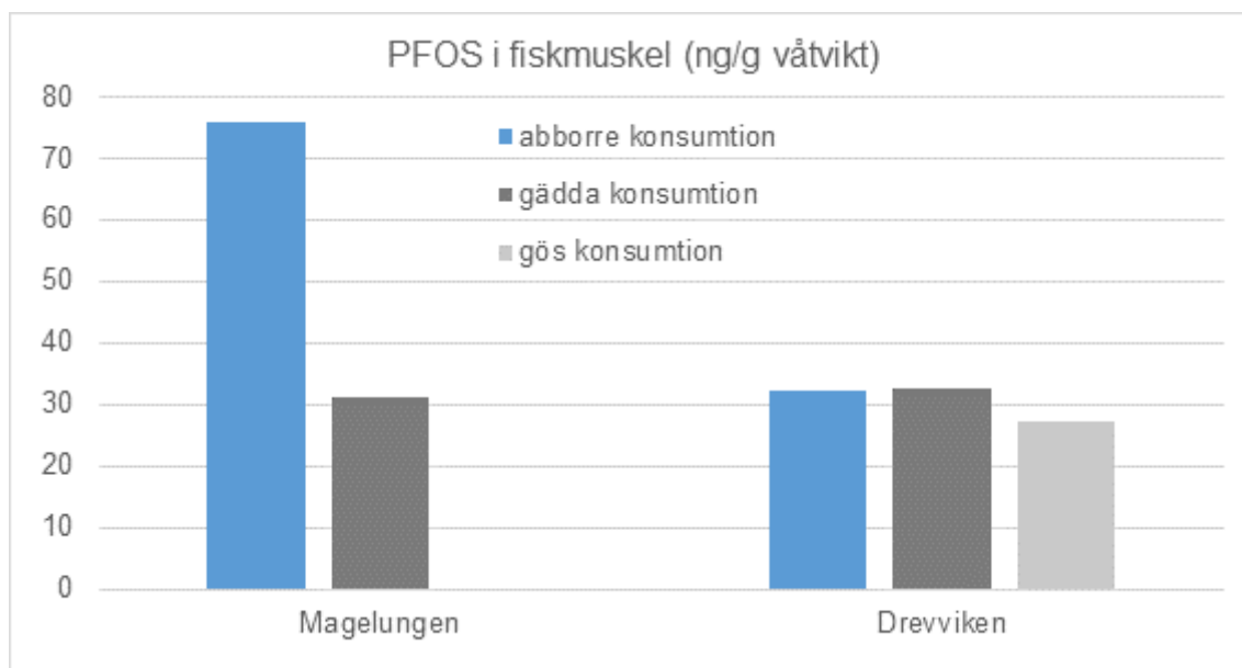
Figur 4. PFOS i muskel från konsumtionsfisk (abborre, gädda och gös) insamlad och analyserad 2021. Diagrammet visar medelvärdet av alla analyserade prov per provlokal (1-4 poolade prov per lokal).
