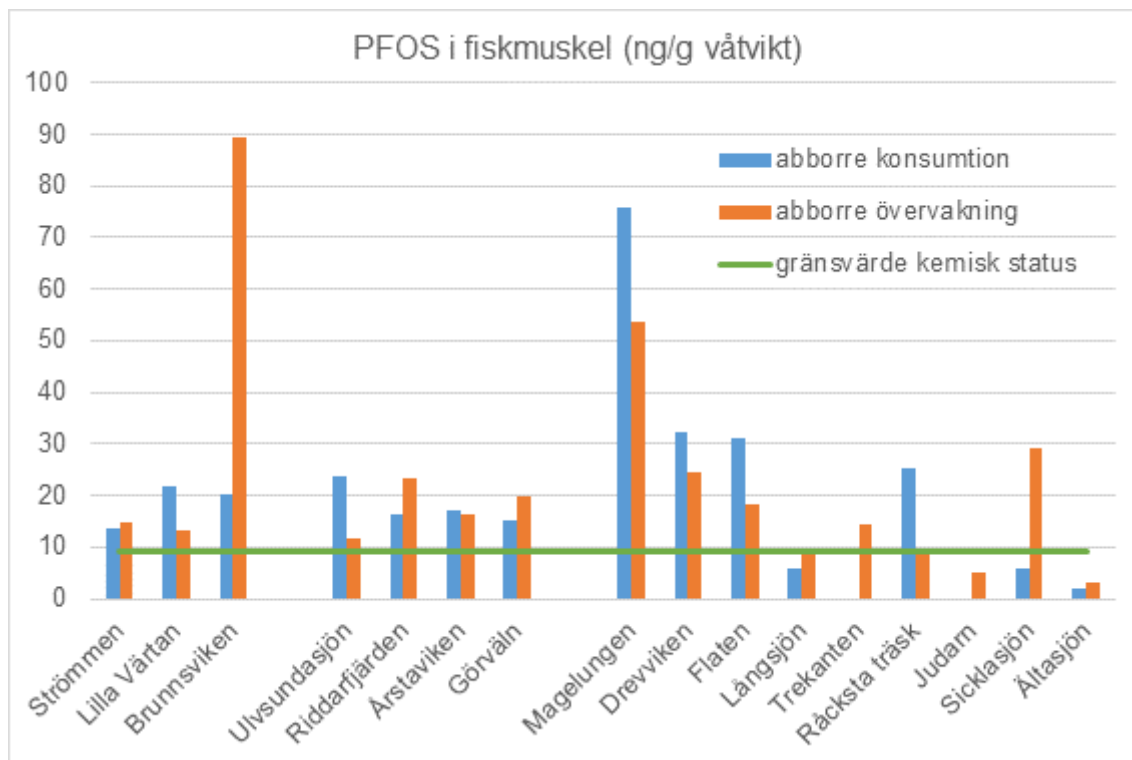
Figur 3. PFOS i muskel från övervakningsabborre och konsumtionsabborre insamlad och analyserad 2021. För övervakningsabborre visar diagrammet halten i ett poolat prov per provlokal. För konsumtionsabborre visar diagrammet medelvärdet av två poolade prov per provlokal. Grön linje visar miljö kvalitetsnormen för PFOS i fisk (9,1 ng/g våtvikt).
