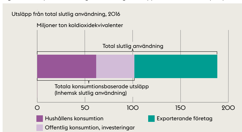
Figur 9.1 Princip för beräkning av växthusgasutsläpp ur ett konsumtionsperspektiv.
