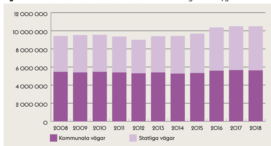
Figur 3.2 Trafikarbete inom Stockholms kommun – vardagsmedeldygn.
