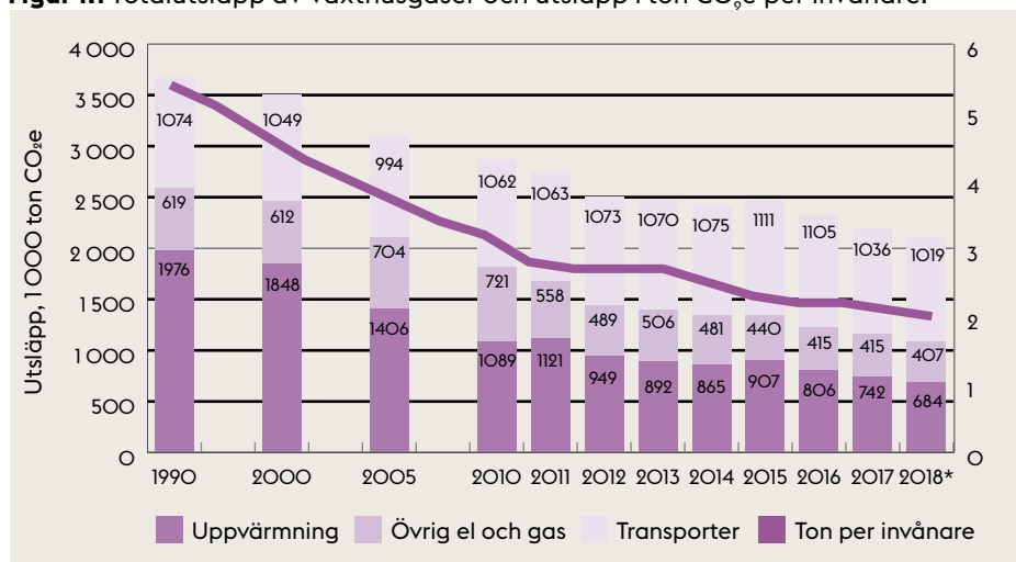
Figur 1.1 Totalutsläpp av växthusgaser och utsläpp i ton CO 2 e per invånare.
