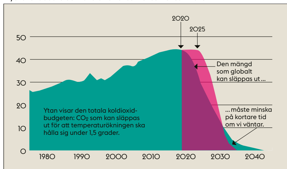
Figur 2.1 Det är den totala mängden växthusgaser i atmosfären som är avgörande för klimatförändringarna. För att undvika temperaturökningar är det därför viktigt att minska de globala utsläppen snabbt redan nu. En senare reduktion måste ske mycket snabbare och får större konsekvenser för samhället.
