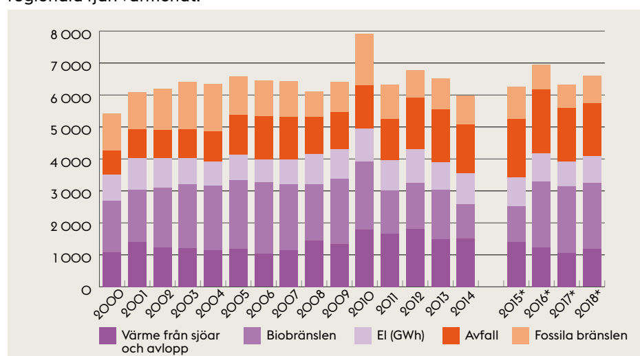
Figur 4.3 Insatta bränslen och energier (ej normalårskorrigerade värden) i fjärrvärmesystem för produktionsanläggningar inom Stockholm stads geografiska gräns 2000–2014, *2015–2018 avser produktionsanläggningar för Stockholm Exergis regionala fjärrvärmenät.
