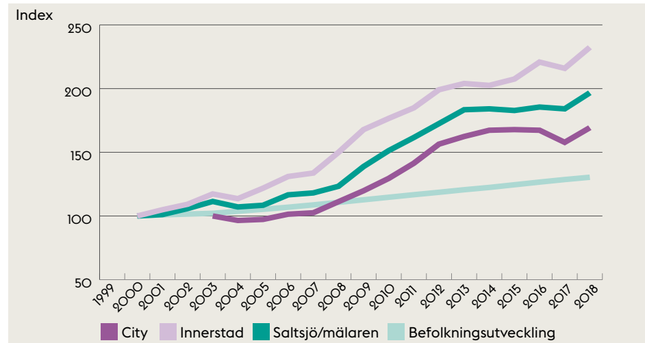
Figur 3.4 Utveckling av cykelpassager per dygn över tre snitt och befolkningsutveckling i länet, 2000–2018, rullande 5 års-siffror, index = år 2000.
