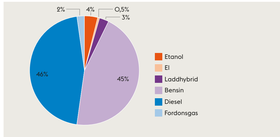
Figur 3.6 Bränslefördelning i Stockholms bilflotta (2017).
