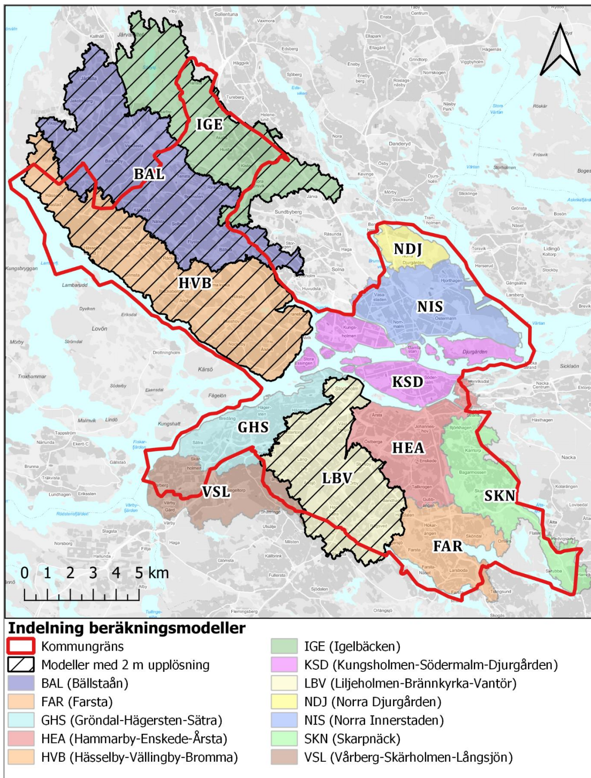
Figur 3. Indelning av Stockholms stad (röd linje) i olika beräkningsområden. Vissa beräkningsområden sträcker sig utanför kommungränser för att få med hela avrinningsområdet och därmed beskriva de översvämningar som kan ske i Stockholms stad. Områden med skrafferade polygoner har 2 m upplösning medan resterande har 1 m upplösning.
