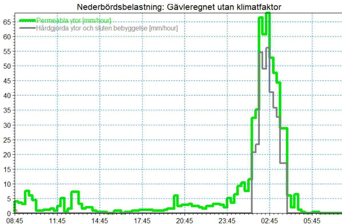
Figur 9: Nederbördsbelastning i skyfallsmodellen för scenariot med det uppmätta Gävleregnet för permeabla ytor (grön linje) samt hårdgjorda ytor och sluten bebyggelse (grå linje).
