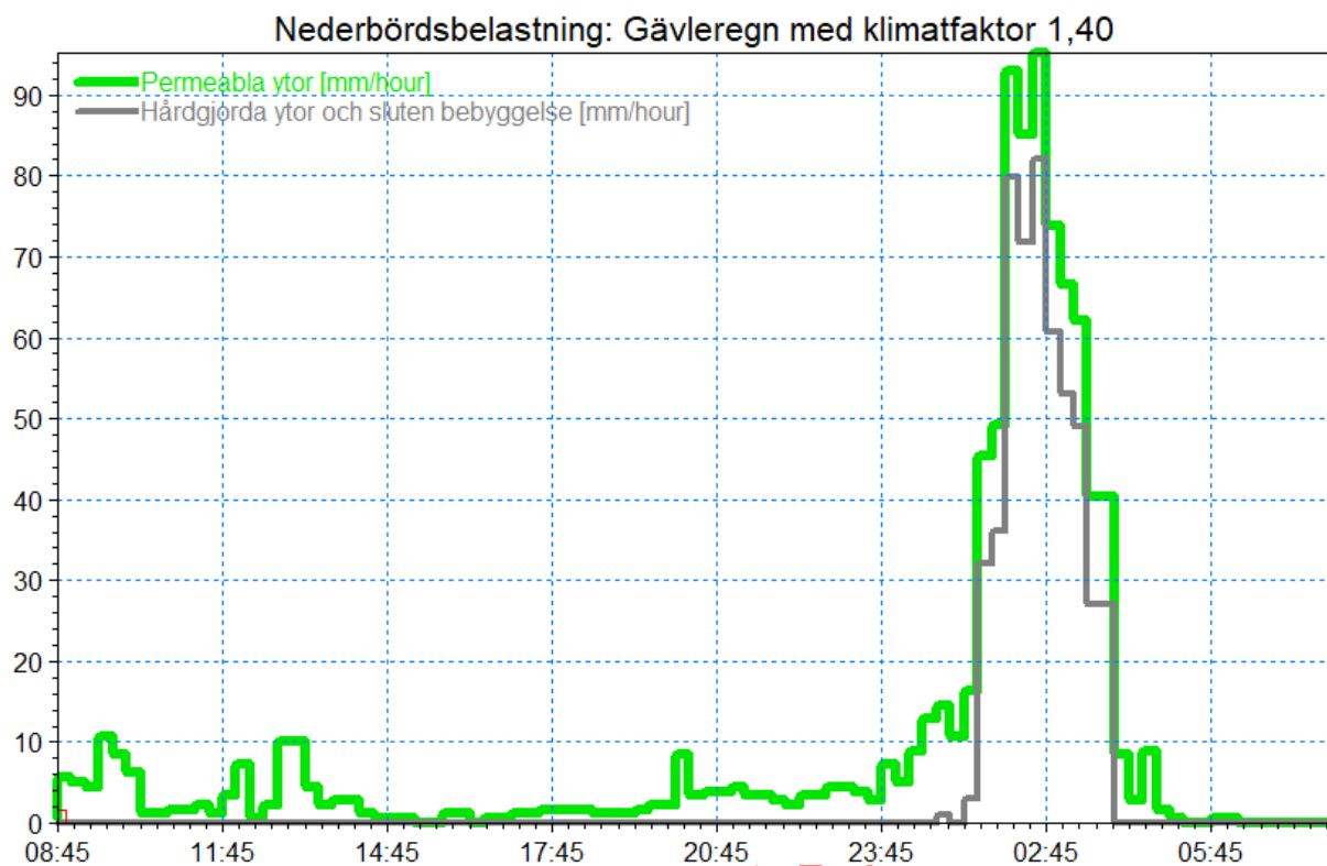
Figur 10. Nederbördsbelastning i skyfallsmodellen för scenariot med det klimatanpassade Gävleregnet för permeabla ytor (grön linje) och hårdgjorda ytor samt sluten bebyggelse (grå linje).
