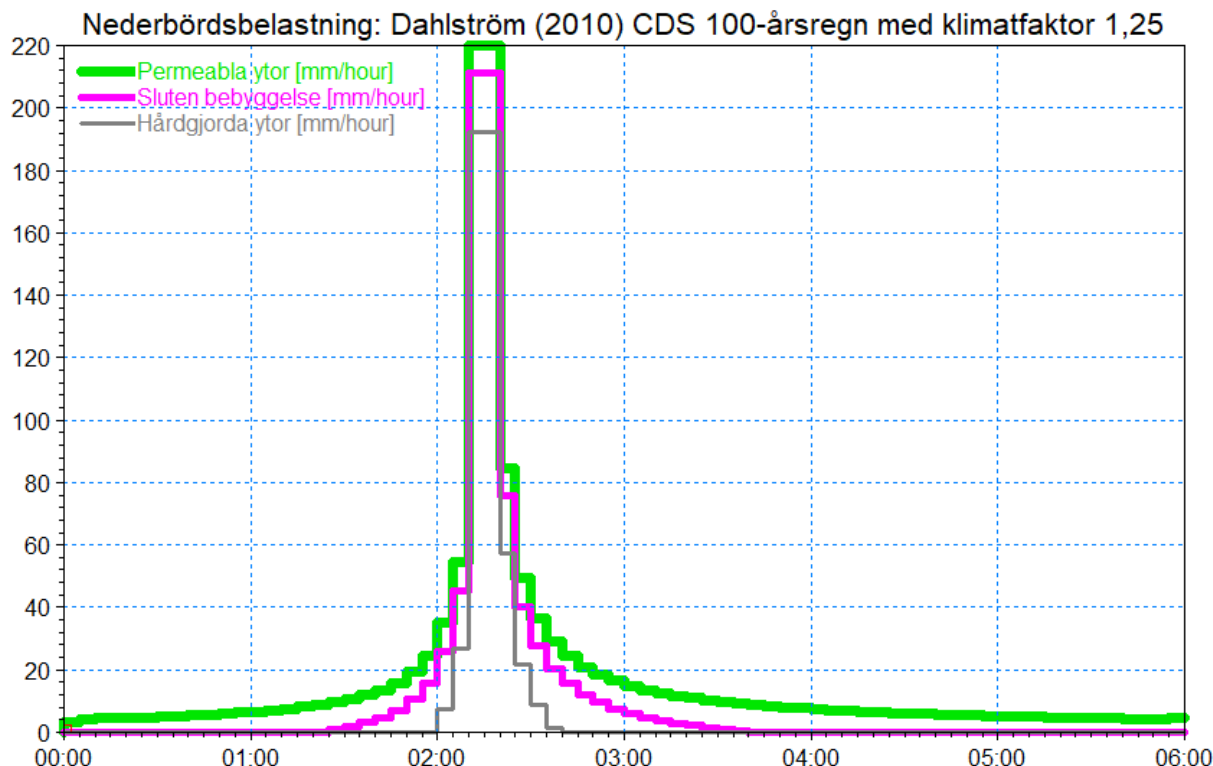
Figur 11: Nederbördsbelastning för scenario Dahlström 2010 CDS 100-årsregn med klimatkfaktor 1,25. Observera att nederbörden pågår i 6 timmar men simuleringen fortsätter ytterligare 2 timmar efter att regnet har upphört.
