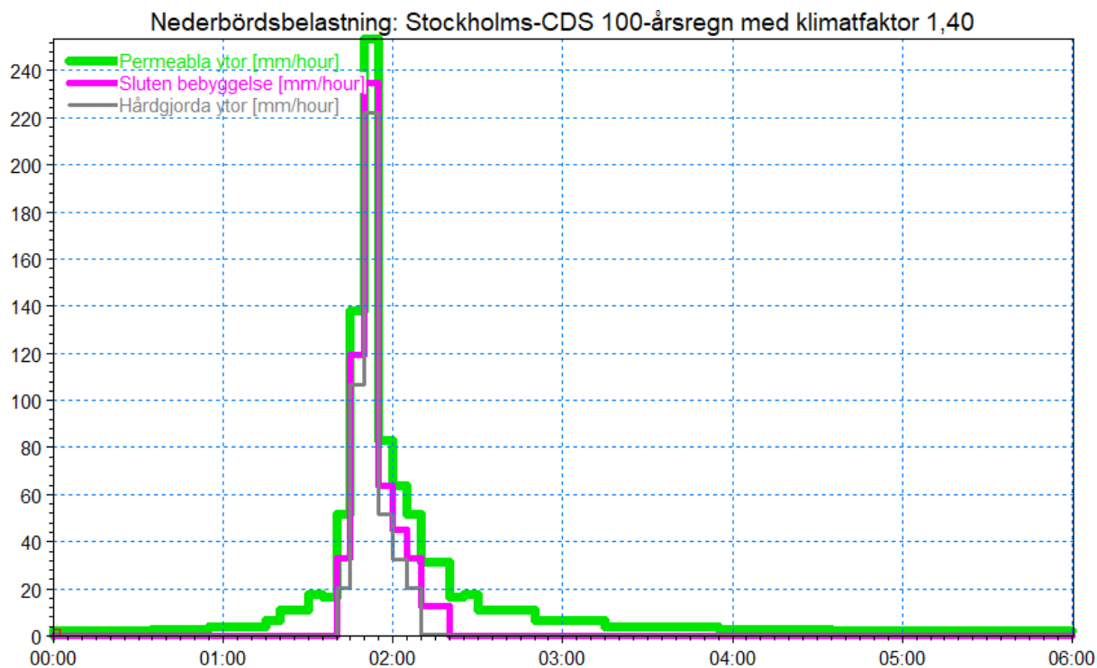
Figur 7: Nederbördsbelastning för scenario Stockholms-CDS 100-årsregn med klimatkfaktor 1,40 och skevhetsfaktor 0,31. Observera att nederbörden pågår i 6 timmar men simuleringen fortsätter ytterligare 2 timmar efter att regnet har upphört.
