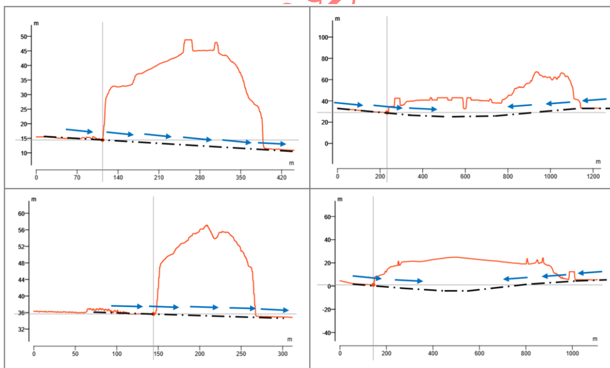
Figur 4. Profil över markhöjder (orange linje) som visar exempel på två tunnlar (streckad svart linje) som lags in som 2D-culverts för att beskriva vattentransport genom tunnelarna (bilderna till vänster.) samt två tunnlar som inte lags in som 2D culverts, eftersom vatten antas ansamlas i lågpunkt inne i tunneln (bilderna till höger).
