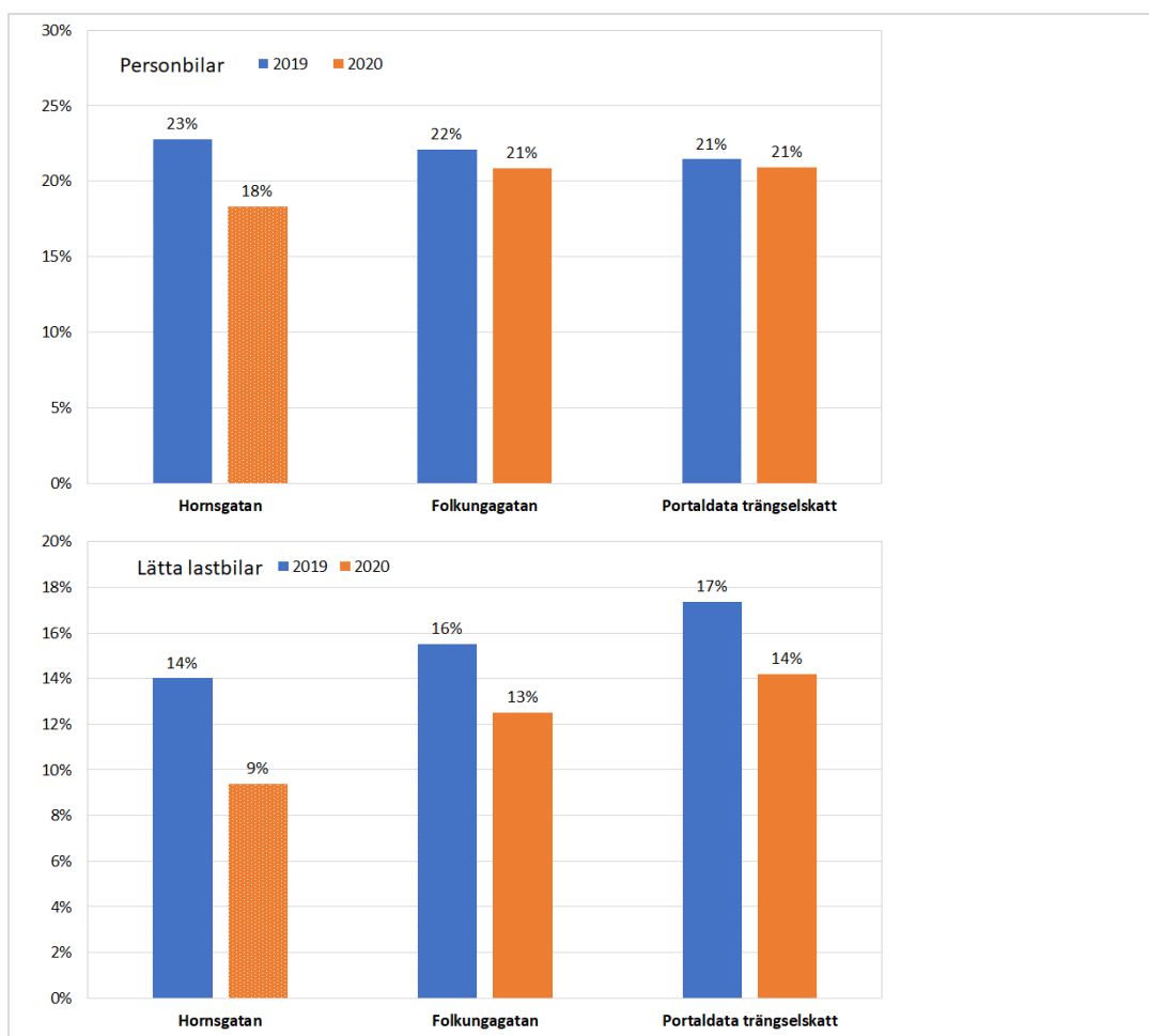
Figur 7. Andelen personbilar och lätta lastbilar med avgaskrav Euro 4 och tidigare klasser. År 2020 i jämförelse med år 2019 på Hornsgatan, Folkungatan och för portaldata för trängselskatt. Euro 4 och tidigare klasser är inte godkända i miljözonen på Hornsgatan år 2020.
