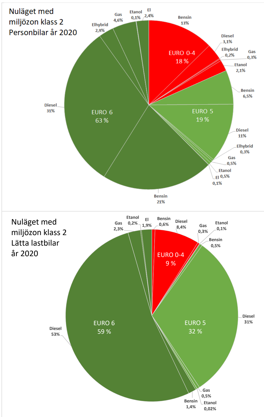
Figur 21. Nuläget, fordonspark år 2020. Uppmått fördelning av godkända (grönt) och icke godkända euroklasser (rött) för personbilar respektive lätta lastbilar med miljözon klass 2 på Hornsgatan. Fördelning på bränslen/drivlinor.
