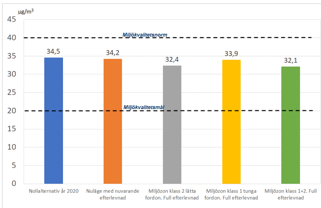
Figur 26. Hornsgatan år 2020. Beräknade halter av kvävedioxid, \text{NO}_2 , (årsmedelvärde) för nollalternativet, nuläget och de olika miljözonalternativen i jämförelse med motsvarande norm- och målvärde till skydd för människors hälsa.
