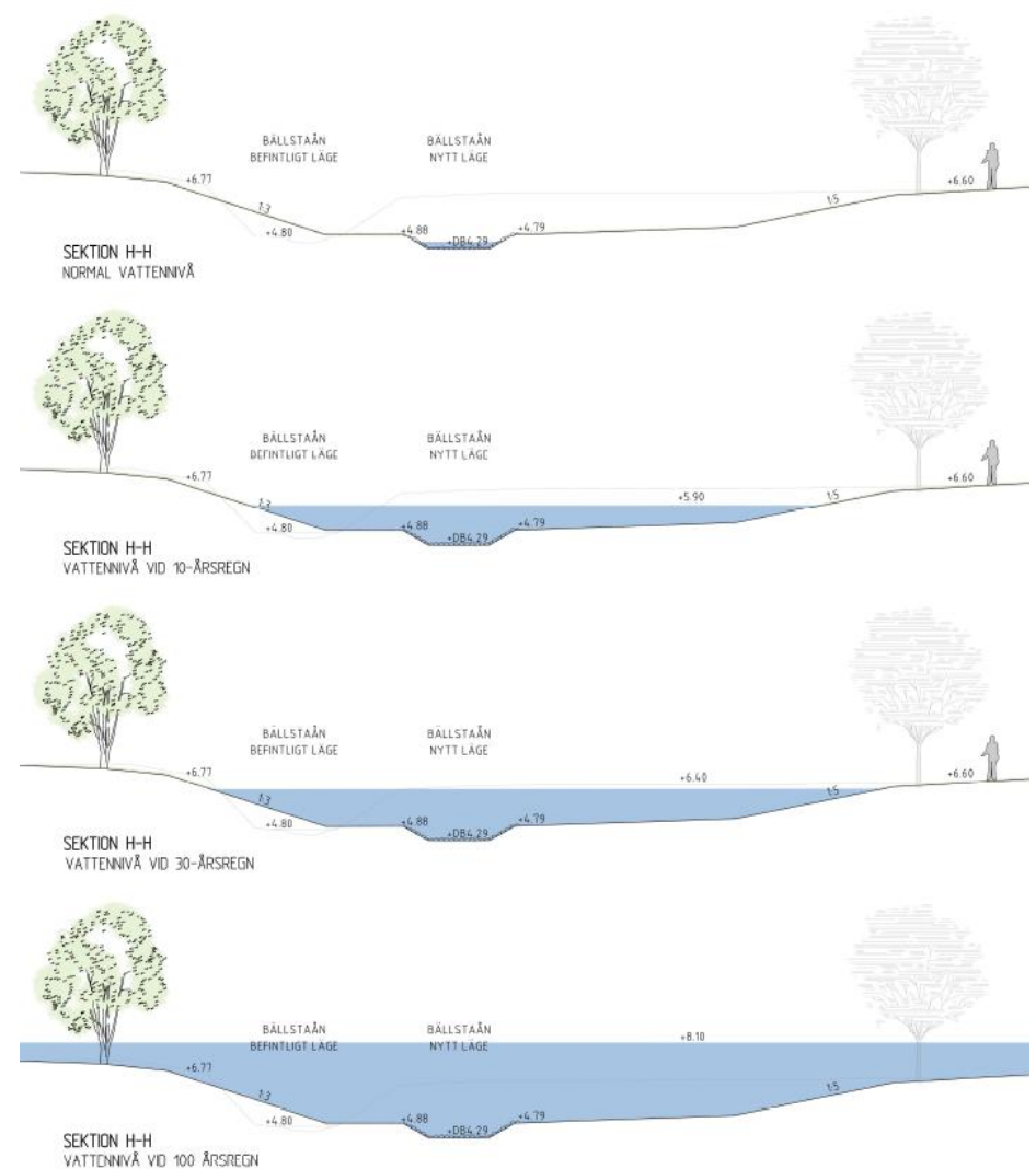
Fig 7. Bällstaåns å-fåra, projekterad lösning med flacka slänter. Översta bilden visar normala flöden, bilden under visar 10-års regn när vattenytan stigit till + 5,90, vid 30-års regn är vattenytan uppe vid +6,40 och vid ett 100-års regn stiger vattnet ytterligare 1,3 m till +8,1. Vid ett sådant 100-års regn kommer stora delar av Tenstadalen stå under vatten (Illustration: Olof Engdahl och Catrin Stengård)
