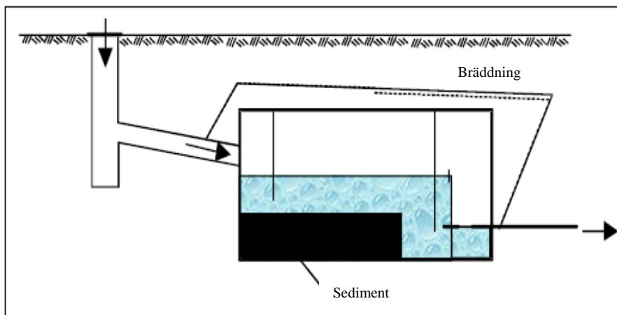
Figur 7: Principskiss över ett avsättningsmagasin. (Bilden är hämtad från rapporten Klassificering av dagvatten och recipienter samt riktlinjer för reningskrav - Rening av dagvatten del 3, Dagvattenstrategi för Stockholm, 2001. )
