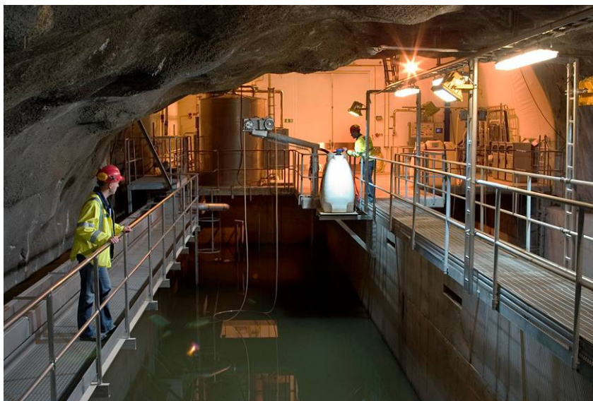
Figur 6: Södra Länkens VA-station. (Vid den borte änden av sedimentationsbassängen syns oljeskimmern samt behållaren med natriumhydroxid.)
