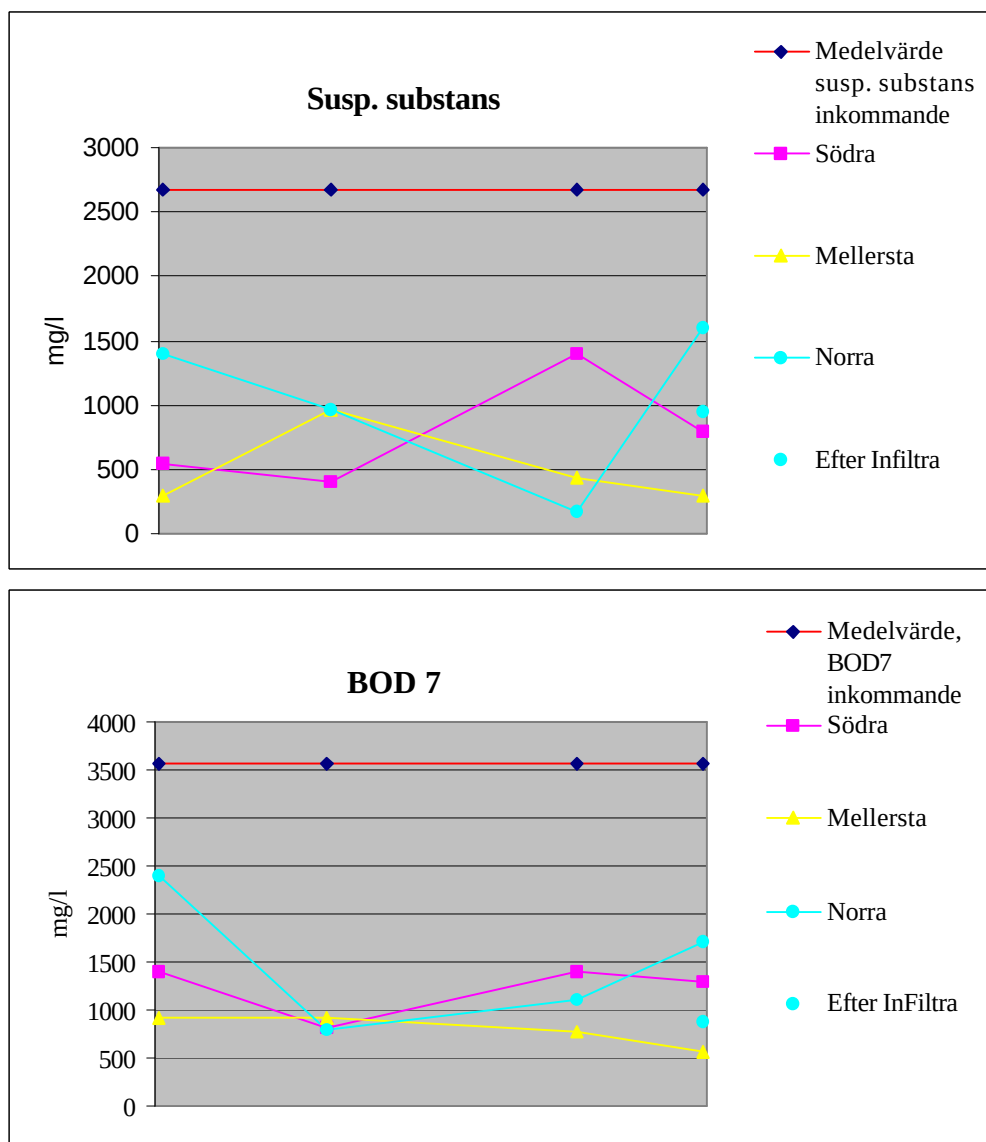
Figur 7. Avskiljning av partiklar (SS) och syreförbrukande ämnen (BOD7) över mullfiltret vid olika provtagningstillfällen maj tom oktober 2007.
