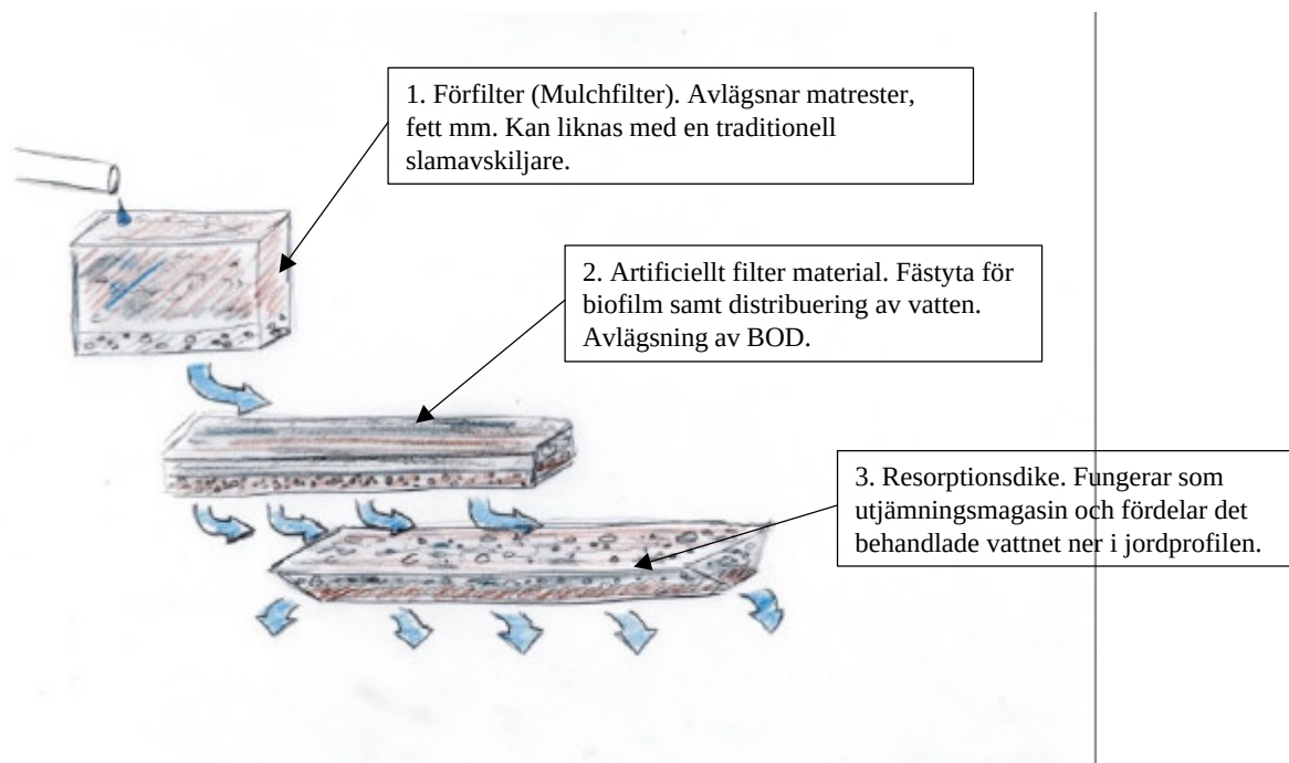
Figur 1 . Processlösningen bygger på behandling och bortledning av vattnet i tre skilda processteg.
