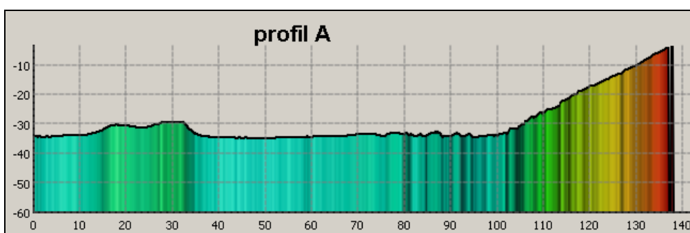
Fig. 19. Profil A genom det centrala skredområdet utanför Lövsta gamla deponiområde. Till höger sprängstensbanken som här har en lutning av ca 38°. Sprängsten förekommer här även ytterligare 20 m utanför släntfoten. För profilens läge se fig. 18.
