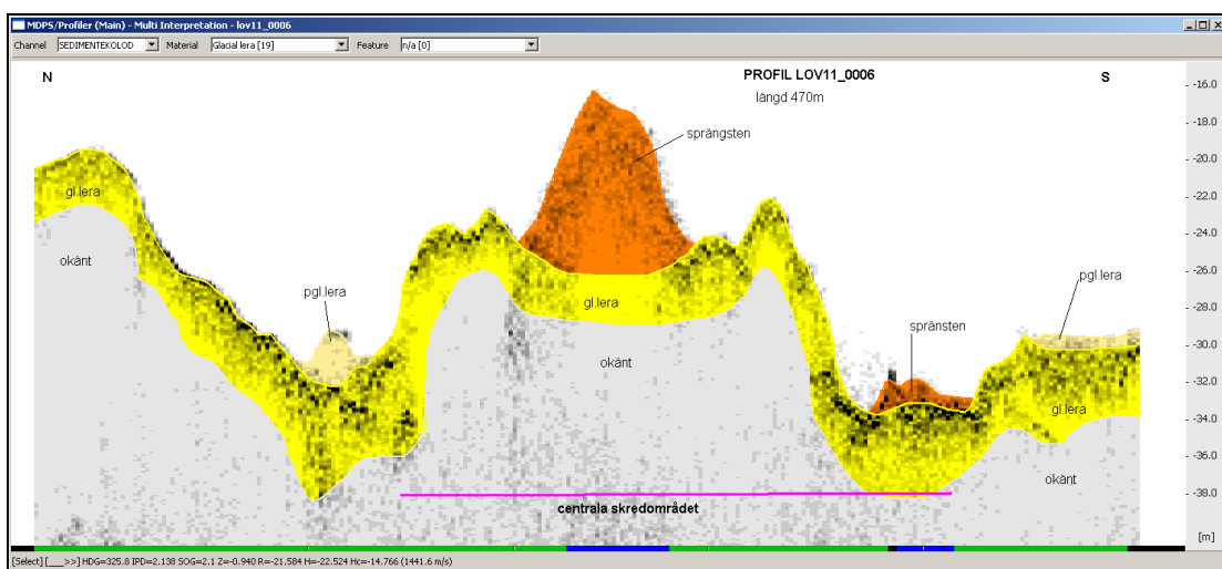
Fig. 22. Sedimentekolodspprofil med tolkning i färg för linje LOV11_0006 löpande utanför Lövsta gamla deponiområde vid Lövstafjärden i Mälaren. För profilens läge, se fig. 13.
