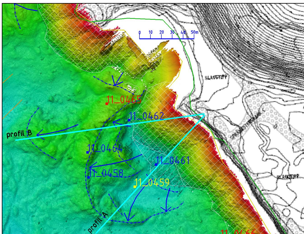
Fig. 18. Terrängmodell över det centrala skredområdet utanför Lövsta gamla deponiområde. Ljusblå linjer markerar läget för profil A och B. Ringmönstrade ytor på landområdet till höger markerar sprängstensbankar som anlades under 1960- och 70-talet för att stabilisera tippen. För teckenförklaring i övrigt se fig. 14.
